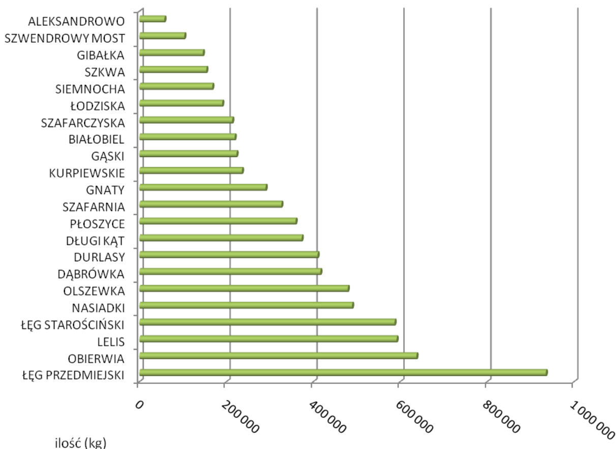
Rysunek 6. Porównanie ilości zinwentaryzowanych wyrobów zawierających azbest dla poszczególnych obrębów ewidencyjnych Gminy Lelis (kg).
